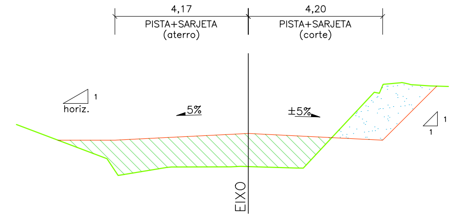
EIXO DA SE-469 EST. 60 a 78
