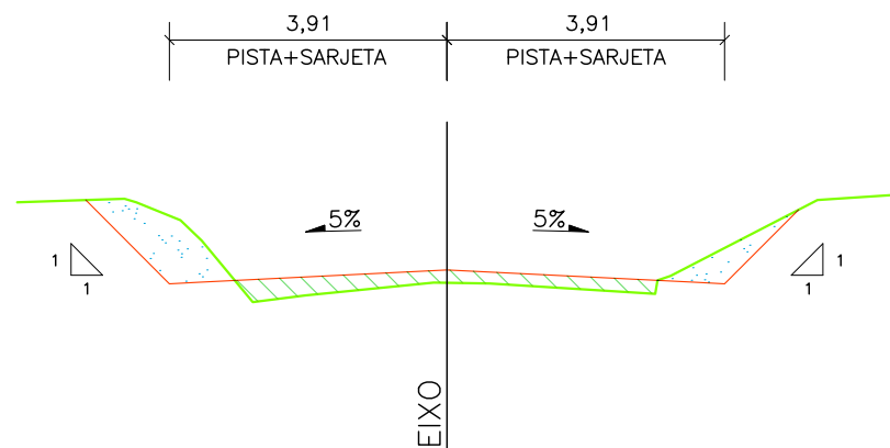
EIXO DA SE-469 EST. 92 a 95 / 106 a 108 / 115 a 138
