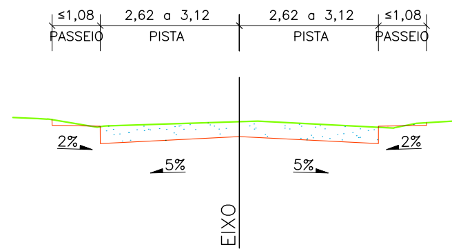
EIXO DA SE-469 EST. 0 a 43 (c/ PASSEIOS)
