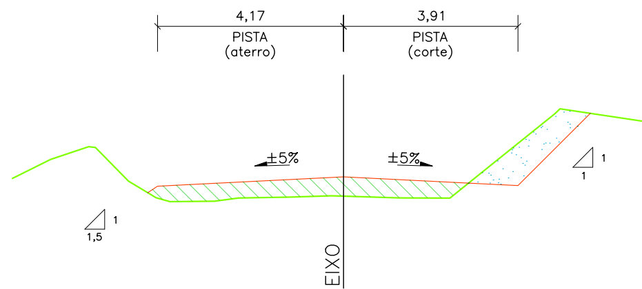
EIXO DA SE-469 EST. 43 a 60 / 78 a 92 / 95 a 106 / 108 a 115 / 138 a 166
